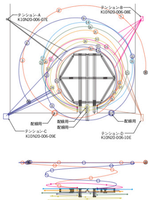
コクーン上部 詳細図 1:60
