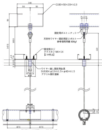
パイプ 詳細図 1:6
