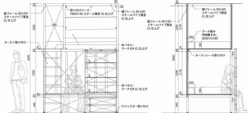
横型ベッド立・断面図 1:40
