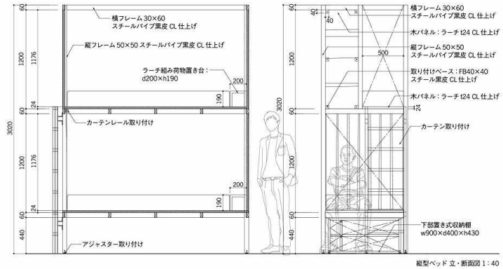
縦型ベッド立・断面図 1:40
