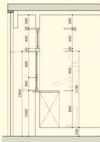
カウンター SECTION 1:50
