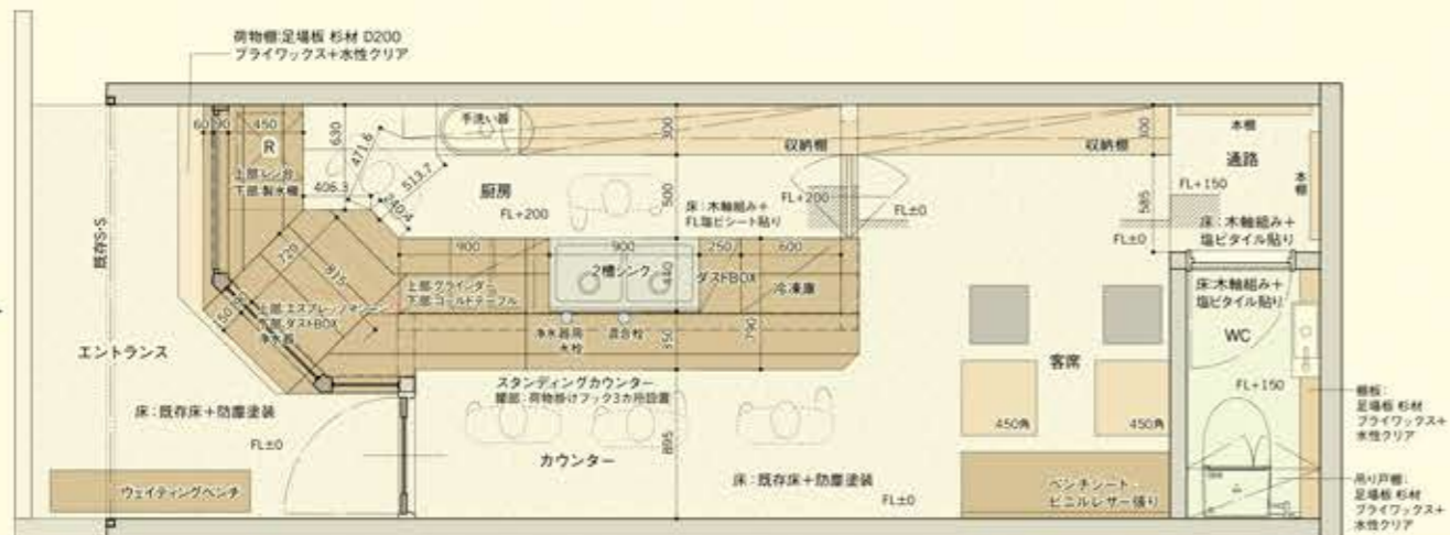
PLAN 1:50
