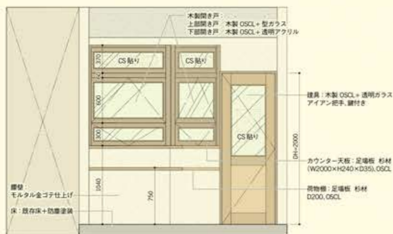
ファサード ELEVATION 1:50
