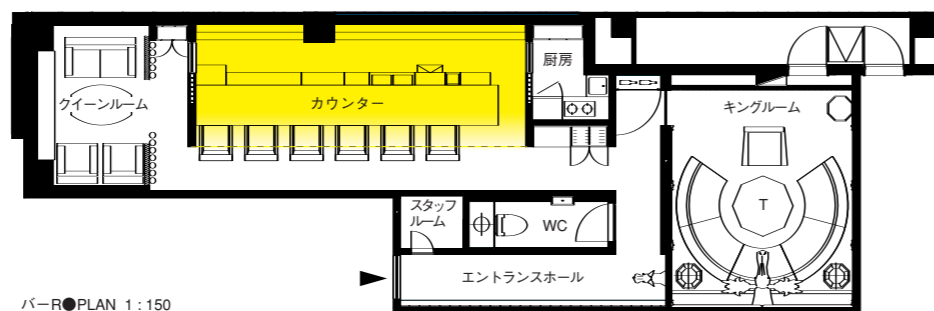
バーR PLAN 1:150
